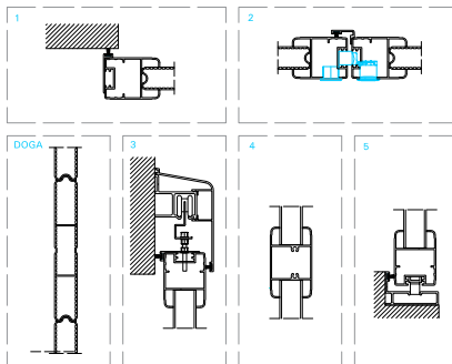
Scurone scorrevole a doghe
