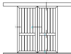
Scurone scorrevole a doghe
