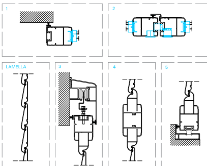
Scurone scorrevole a lamelle
